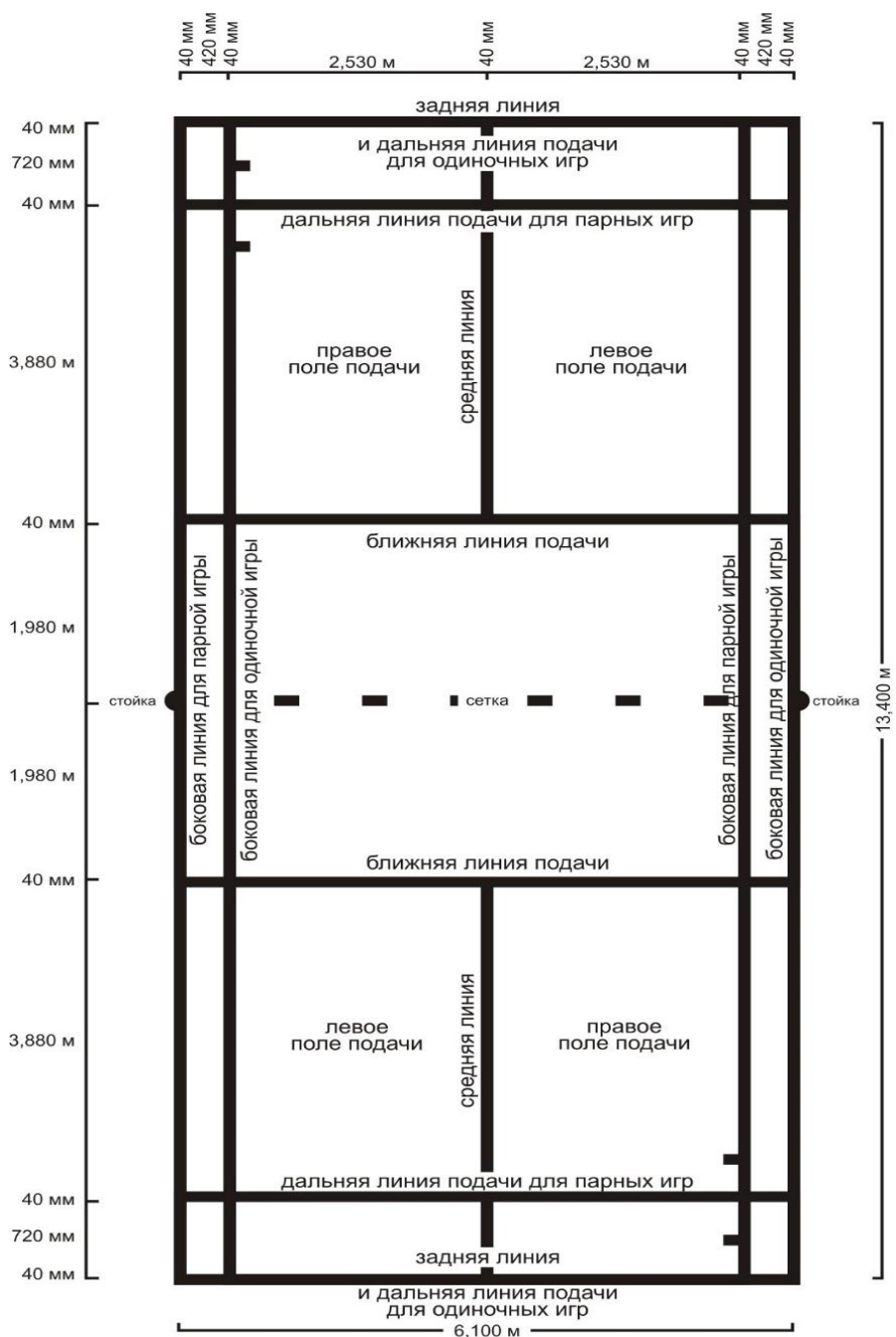
Рис. 1. Разметка корта для парной и одиночной игры. Примечание: Длина корта (площадки) по диагонали –14.723 м.
